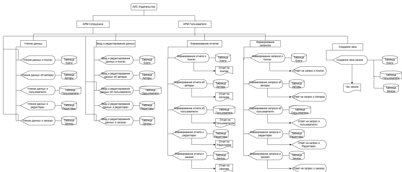
Лист 7. Структурная схема работы системы.
