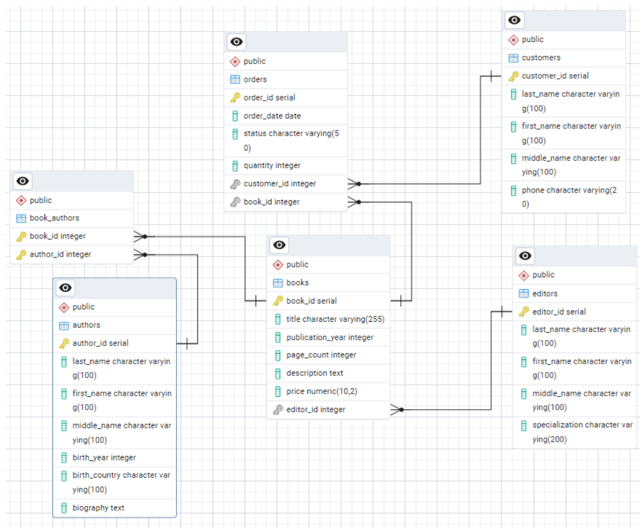
Лист 5. Даталогическая модель предметной области.
