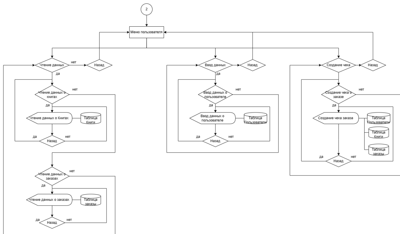
Лист 7. Структурная схема работы системы.
