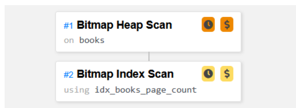
Рисунок 16 – Анализ оптимизированного запроса
