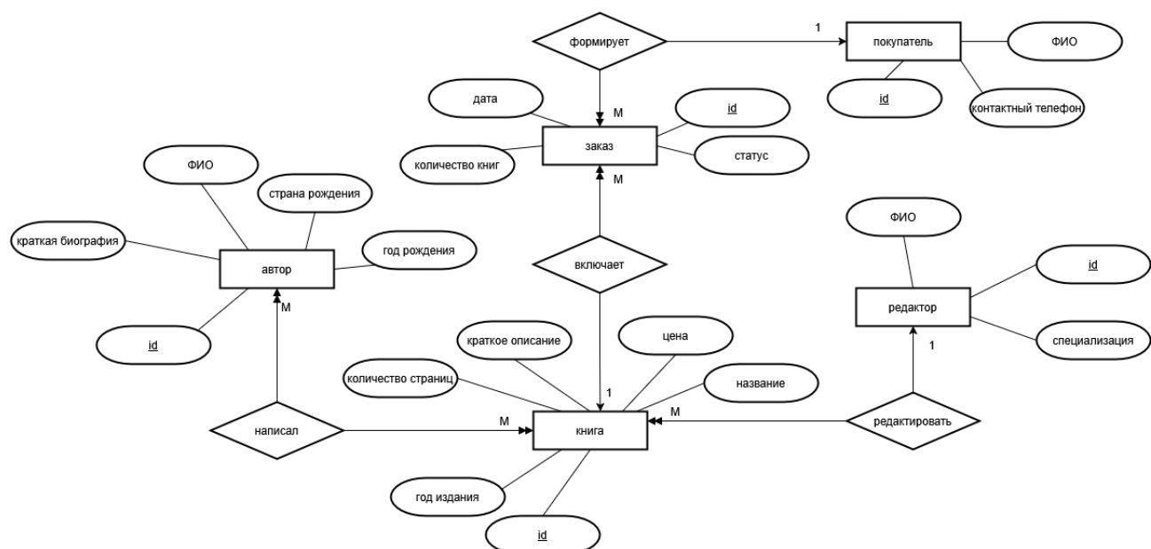
Лист 5. Даталогическая модель предметной области.
